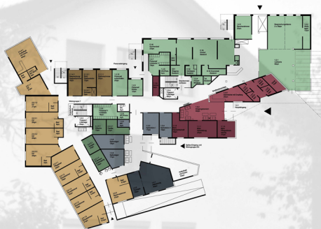
GRUNDRISS ERDGESCHOSS
