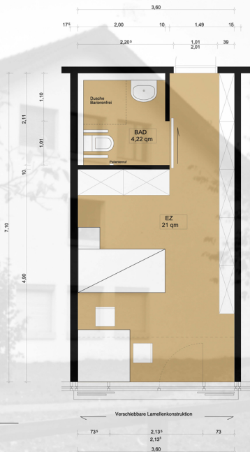
GRUNDRISS REGELZIMMER
